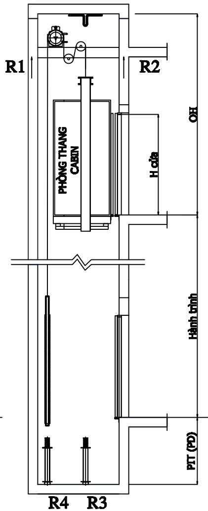
Thang không phòng máy
